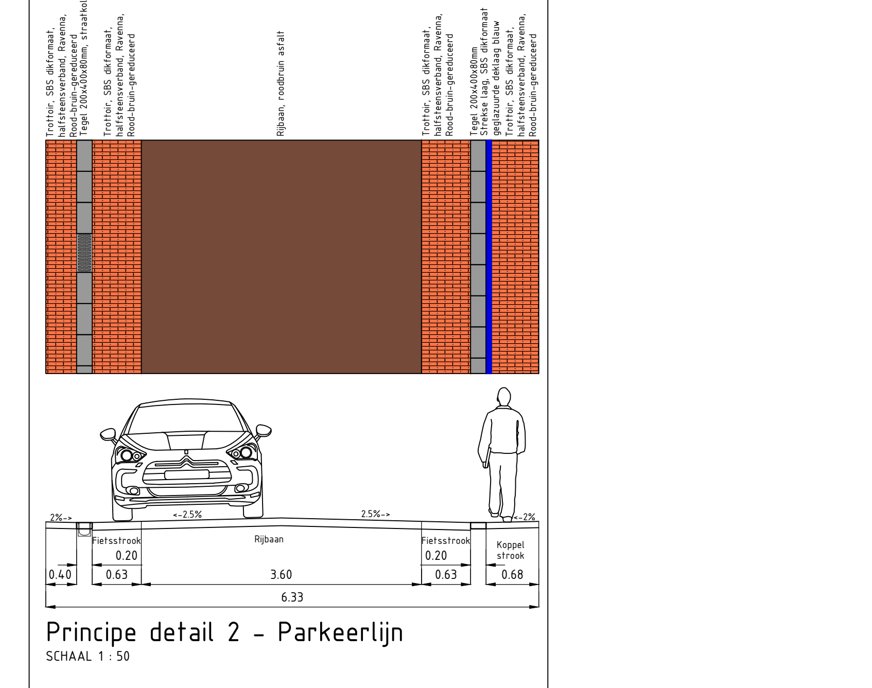
Principe detail 2 - Parkeerlijn SCHAAL 1:50
