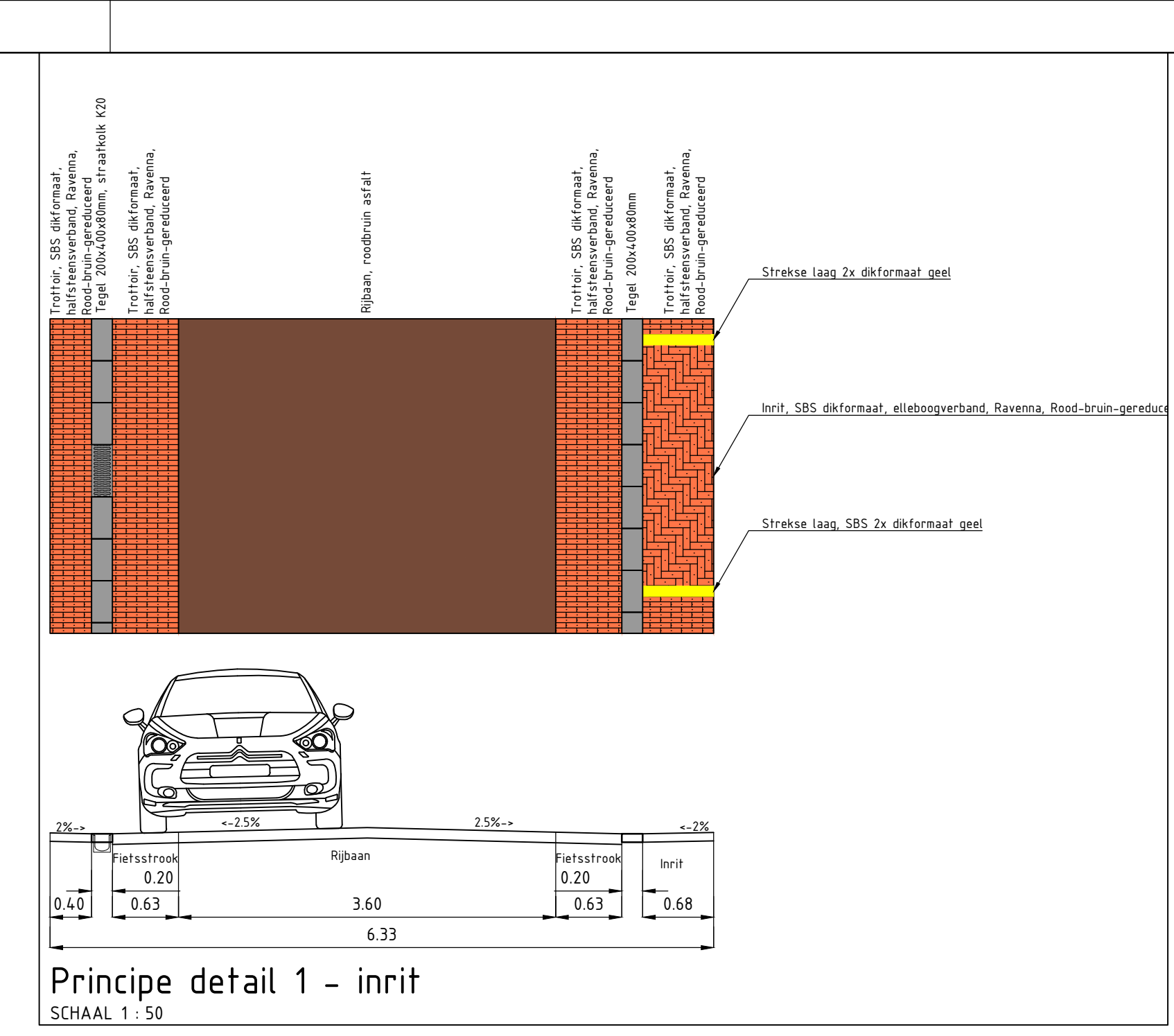
Principe detail 1 - Inrit SCHAAL 1:50
