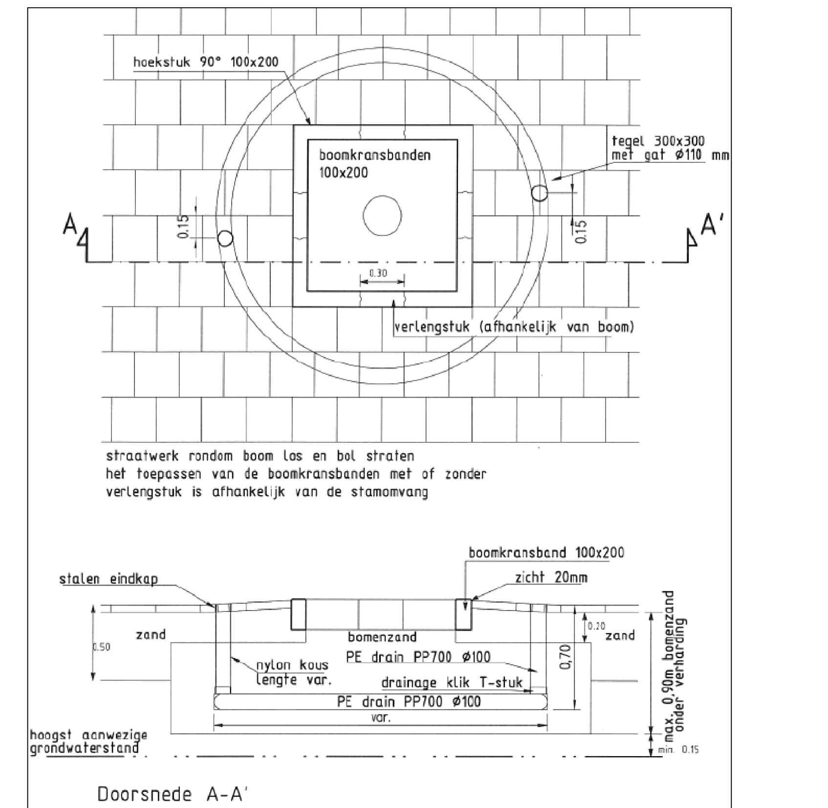
Principe detail 5 - Boomvak Conform Handboek Gemeente Papendrecht (tekeningnummer 5.01)
